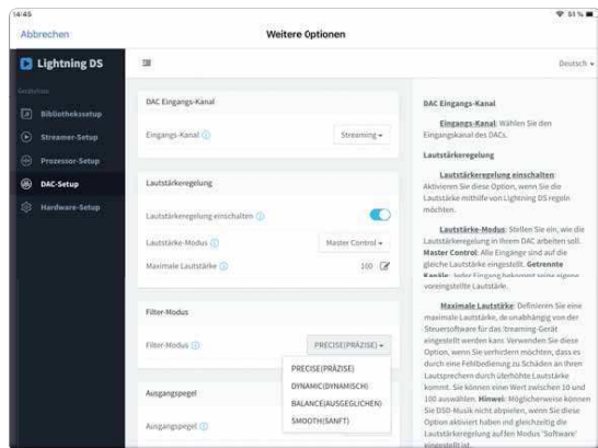
Das Webmenü des Altair wird direkt aus der App heraus aufgerufen und ermöglicht so das Einstellen von Upsampling und Filtern
